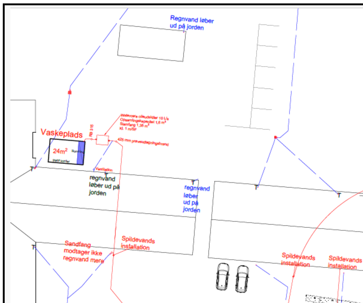
Afløbsplan for virksomhedens vaskeplads
