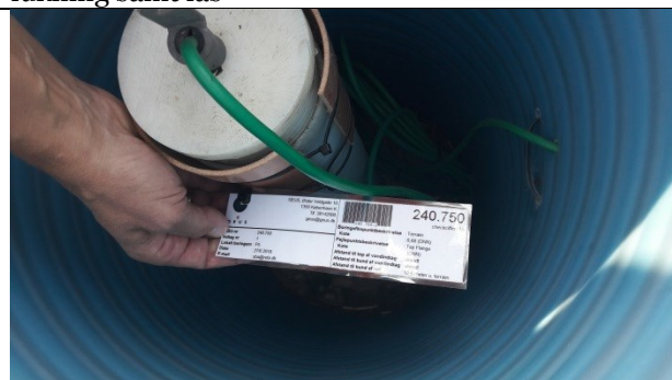
P5 – perkolatpejlebrønd midt i deponiet
