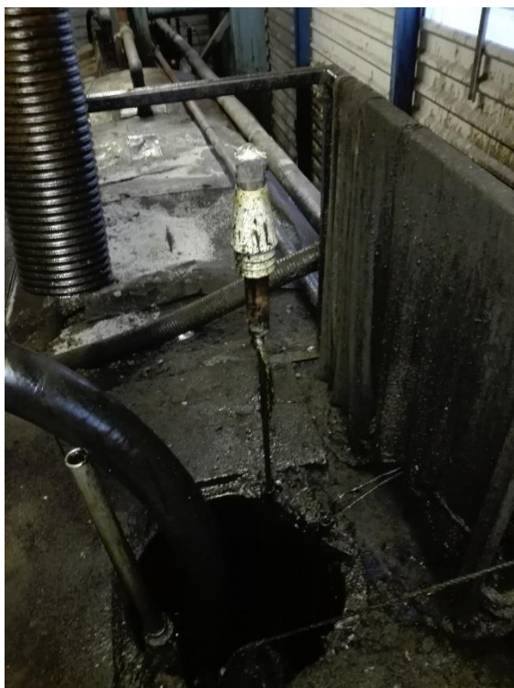
Pejeanordning i modtagetank. Billede heraf kan sendes til telefon.
