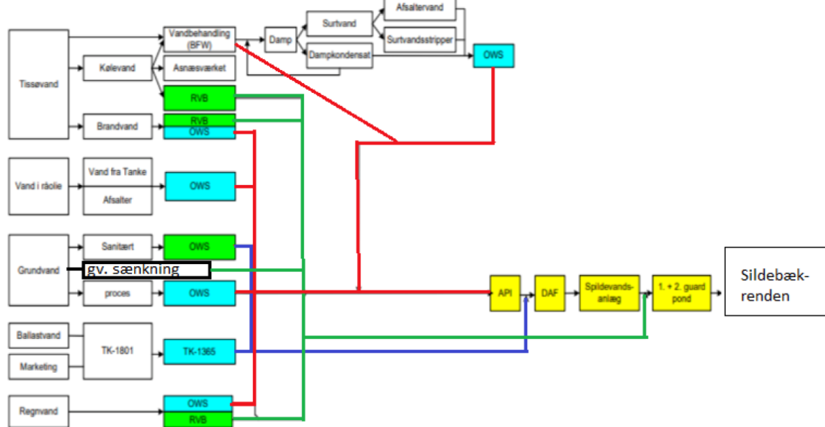
Figur 3.5 Principskitse af spildevandsstrømme, der udledes via Guard Pond 2 og til Sildebækrenden. OWS angiver oliekloak og RVB angiver rentvandskloak. Oliekloak indeholder industrielt belastet overfladevand, ballastvand og slop-olie fra tankskibe, rengøringsvand fra Marketing/Terminalen, brandslukningsvand og spildevand fra afsalter, surtvandsstripper og dampkondensat som oprindelig var Tissøvand. Til RVB løber ubrugt brandvand (Tissøvand),
