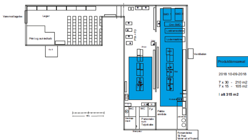
Figur 1 Indretningsplan - Industrivej 4
