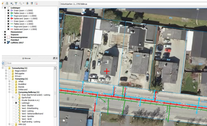
Figur 1 Forsynings ledninger i området
