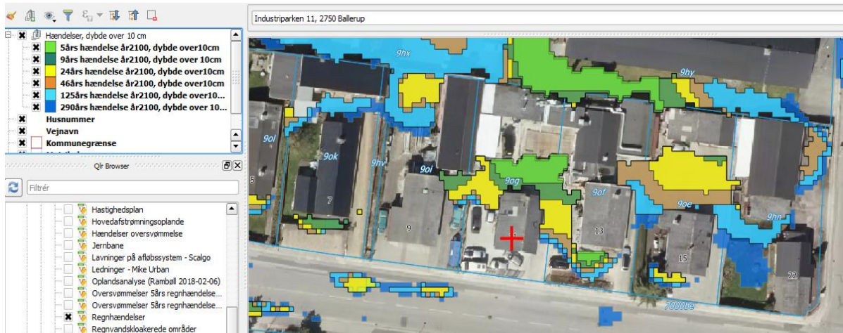
Figur 3 Regnhypigheder der giver oversvømmelse med mere end 10 cm vand på terræn
