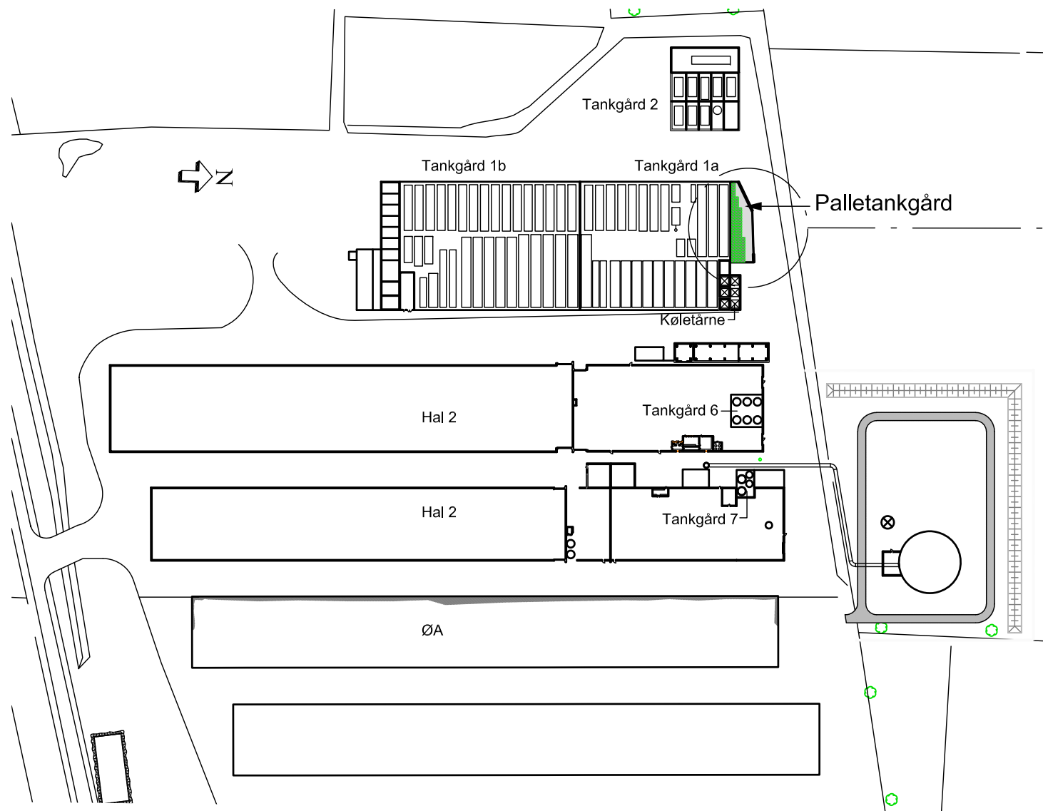
Oversigtsplan Mål 1:2000
