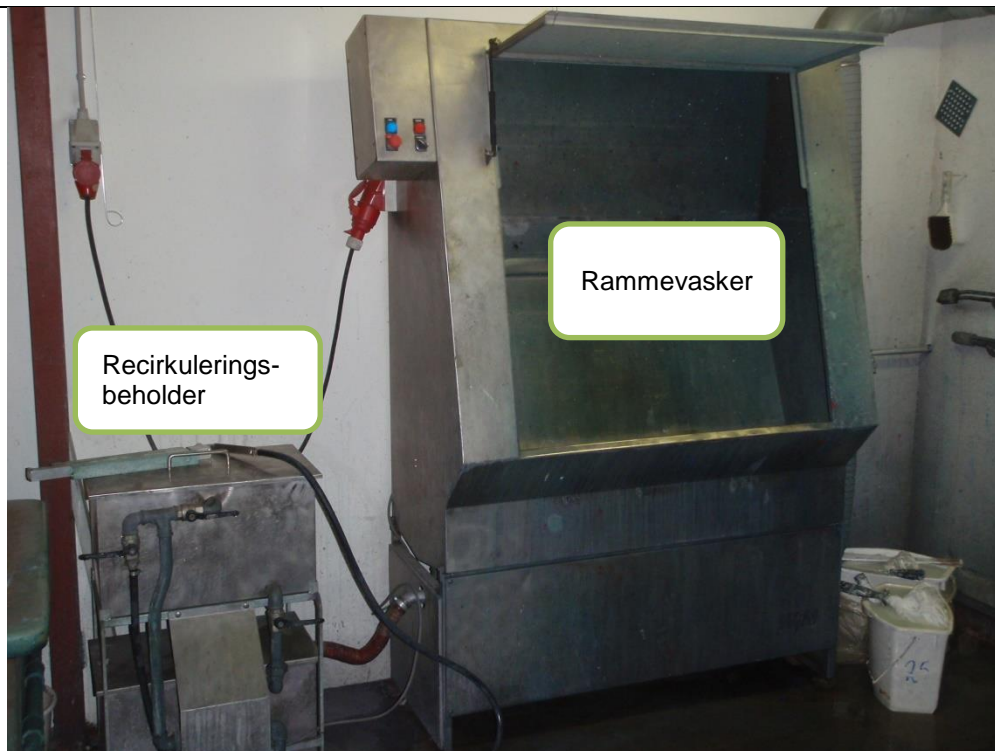
Rammevasker med recirkuleringsbeholder til PN-rammevask ved siden af (billede fra tilsyn i 2012).
