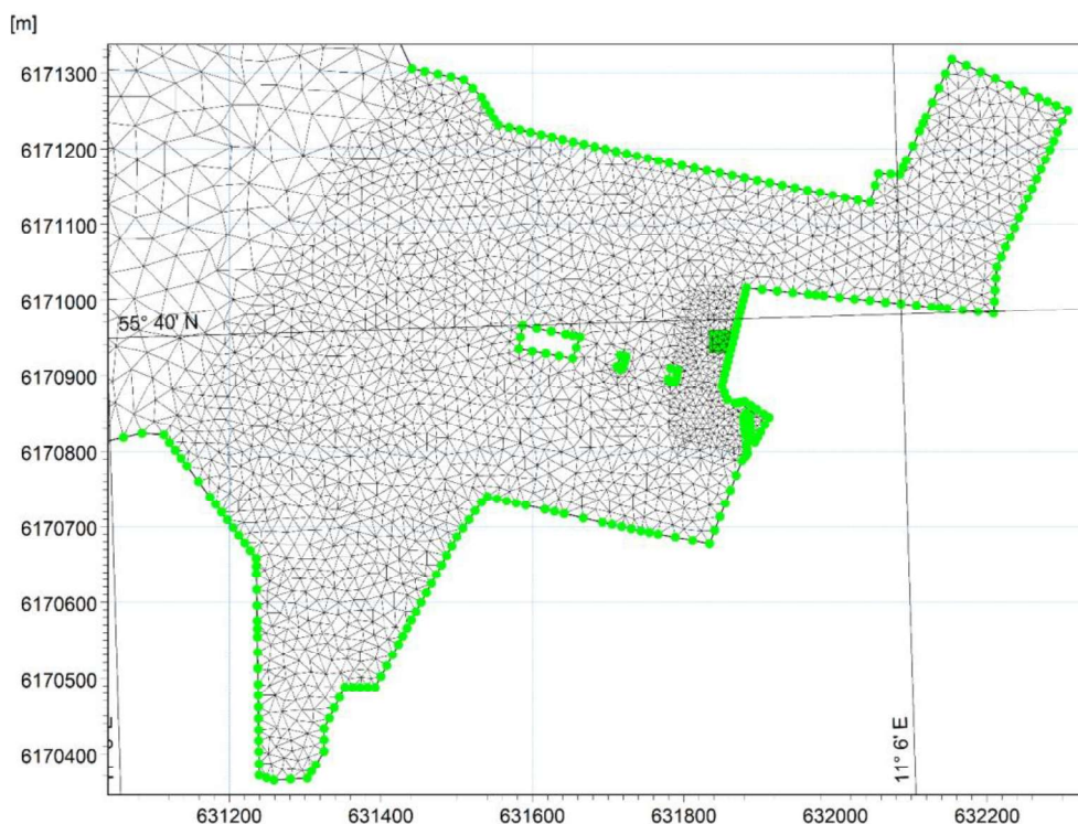
Figur 2.2: Beregningsnet af Kalundborg Havn omkring oliepiere, som udgør nærfeltet omkring udløbspunktet. Udløbspunktet er vist med grøn firkant.
