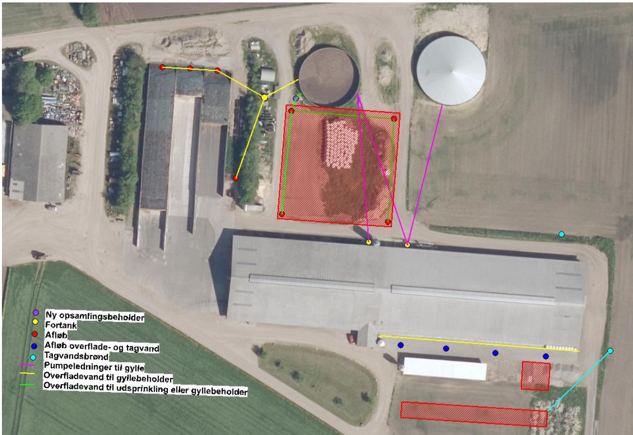
Figur 3. Afløbsplan
