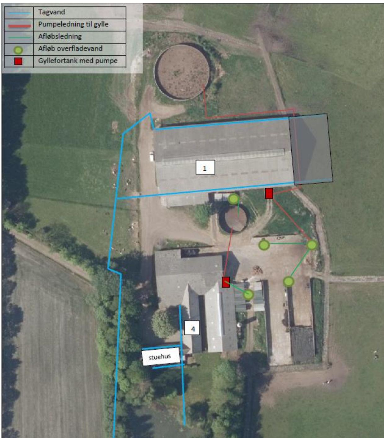
Figur 4. Afløbsplan.
