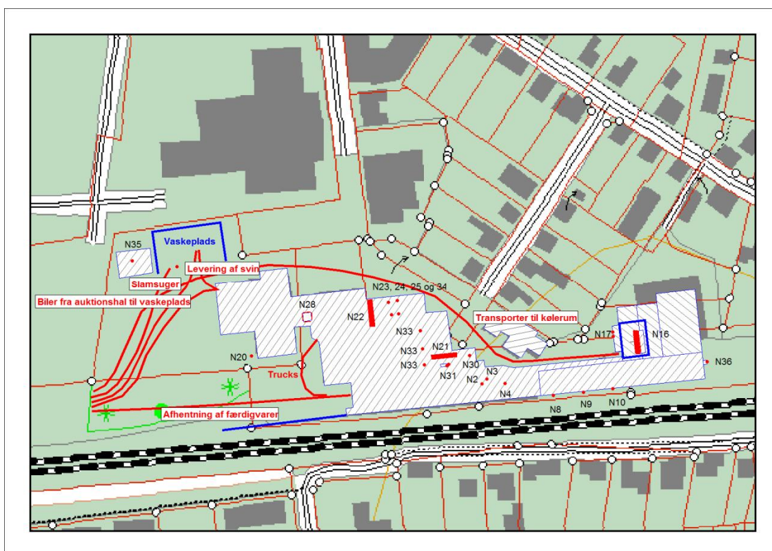
Figur 1: Støjkliddeplacering.
